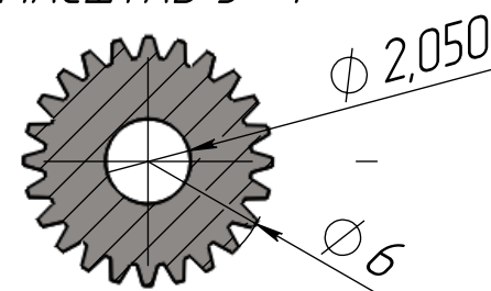
СЕЧЕНИЕ А МАСШТАБ 5 : 1
